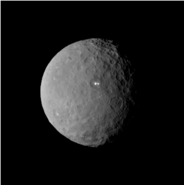
Cérès à 46000 km – Crédit NASA/JPL-Caltech/UCLA/MPS/DLR/IDA
